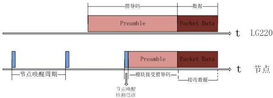
图 15 轮询唤醒模式时序
